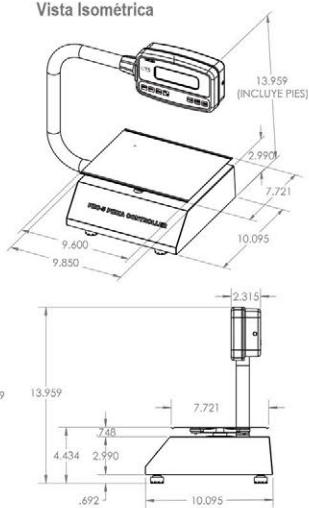
Vista Lateral
